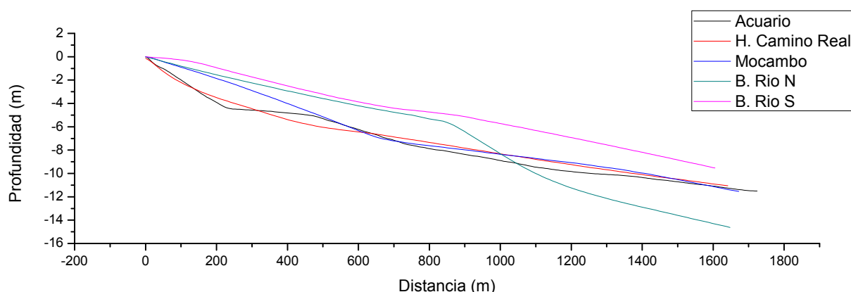
Figura 8. Perfiles batimétricos de la línea de costa hacia mar adentro, en el destino turístico de Veracruz
