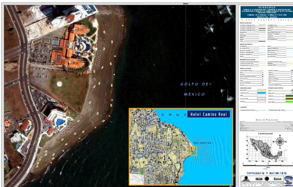
Figura 4. Topografía de la playa frente al Hotel Camino Real en el destino turístico de Veracruz
