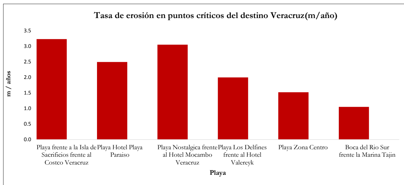
Figura 15. Tasa de erosión en puntos críticos del destino turístico de Veracruz
