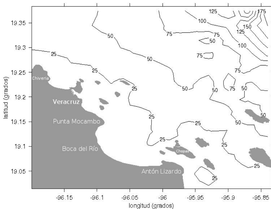
Figura 9. Batimetría de la zona de estudio en Veracruz
