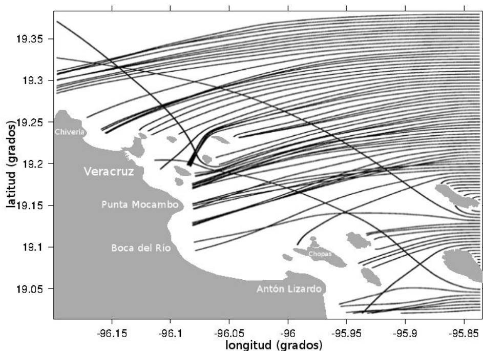
Figura 20. Comportamiento de ortogonales de oleaje en Veracruz, provenientes de la dirección E, con periodo de 20 segundos, asociado a huracanes
