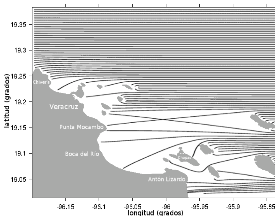
Figura 19. Comportamiento de ortogonales de oleaje más frecuente en Veracruz, provenientes de la dirección E, con periodo de 7 segundos
