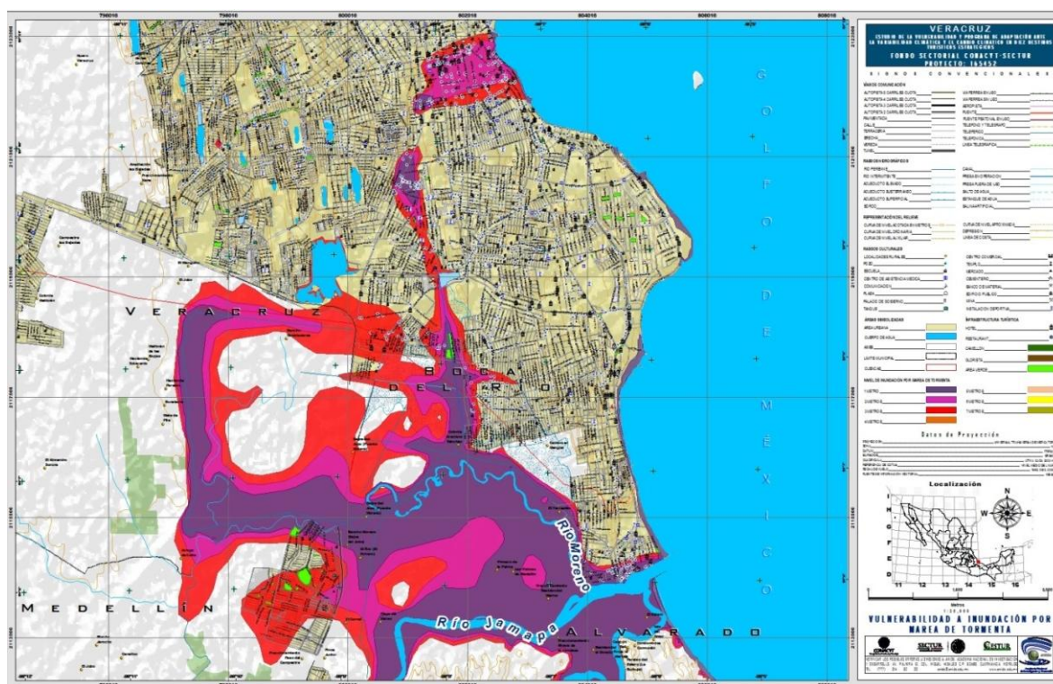
Figura 18. Zonas vulnerables a inundación por marea de tormenta en el destino turístico Veracruz
