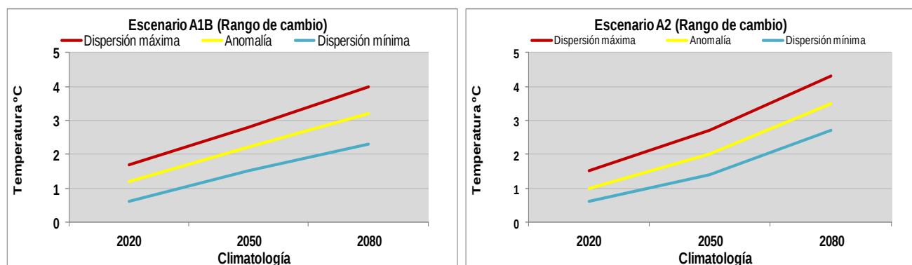
Figura 11. Cambio de Temperatura Media Anual (°C) para diferentes años en Los Cabos.
