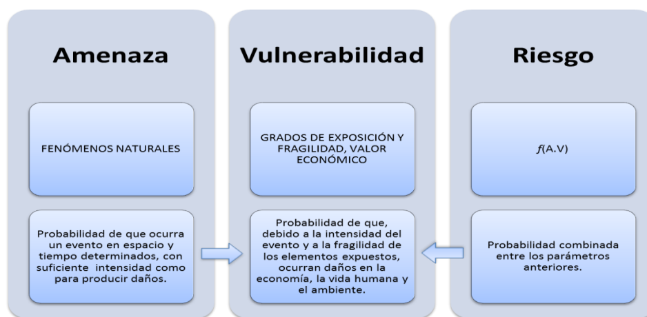
Figura 32. Esquema de los conceptos asociados al riesgo.
