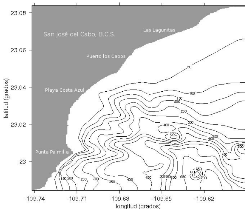
Figura 7. Batimetría de San José del Cabo, Los Cabos
