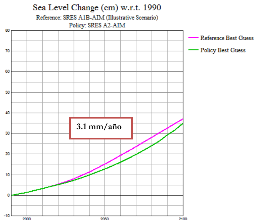
Figura 13. Gráfica del cambio del nivel del mar en cm, de 1990 a 2100
