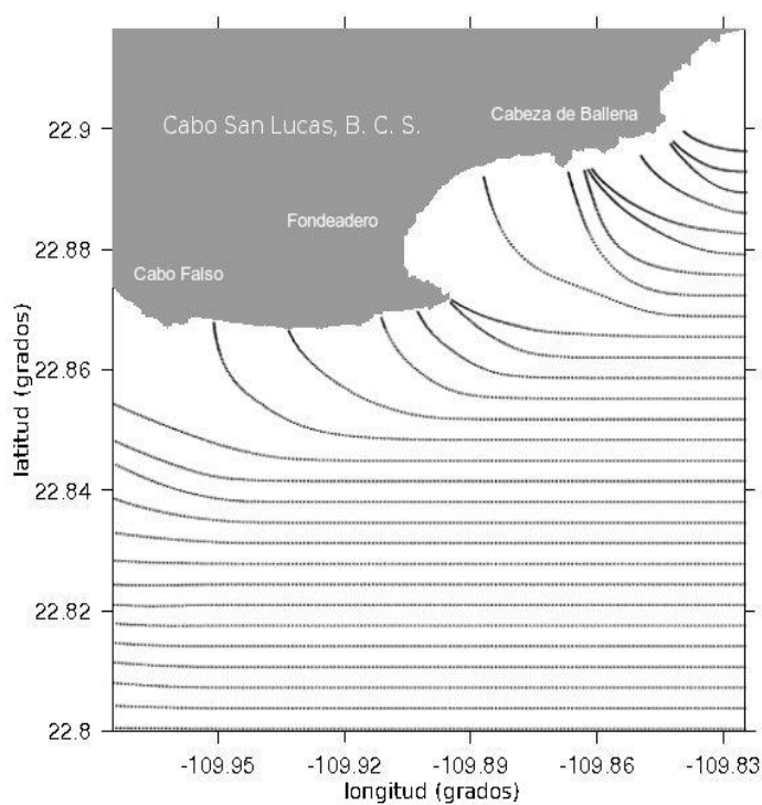
Figura 24. Comportamiento de ortogonales de oleaje en Cabo San Lucas, provenientes de la dirección E con
