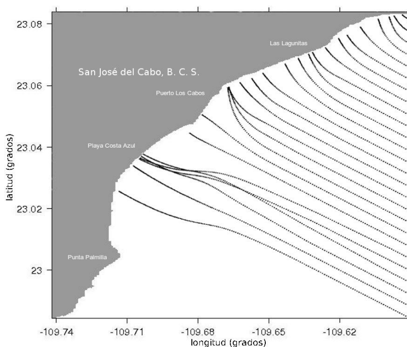
Figura 23. Comportamiento de ortogonales de oleaje en San José de Cabo, provenientes de la dirección ESE con periodo de 22 segundos
