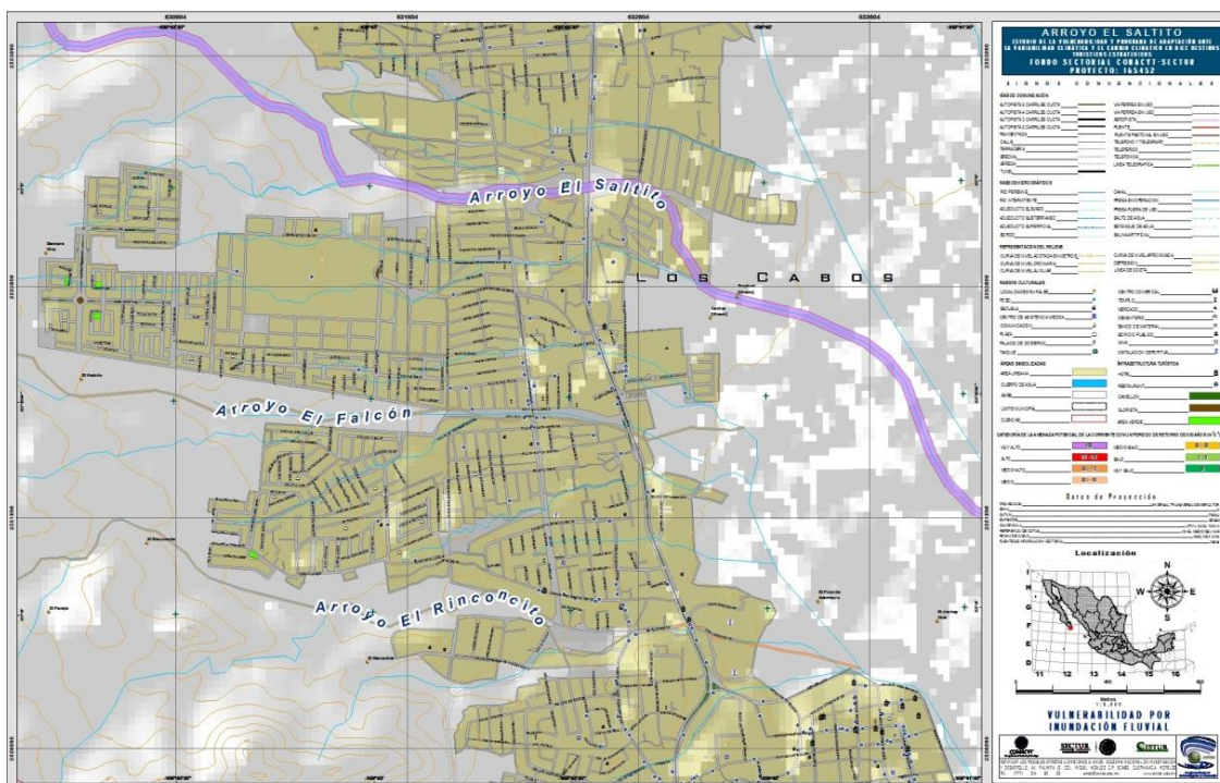
Figura 28. Áreas de inundación fluvial del río El Saltillo en el destino turístico de Los Cabos
