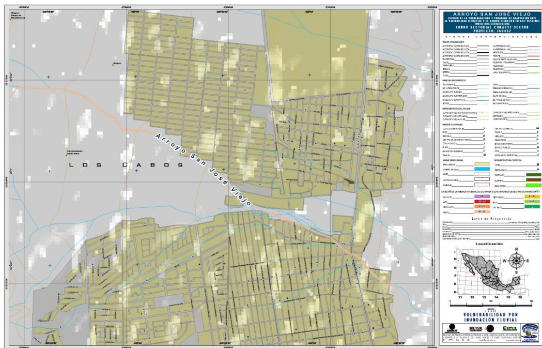
Figura 31. Áreas de inundación fluvial del río San José Viejo en el destino turístico de Los Cabos
