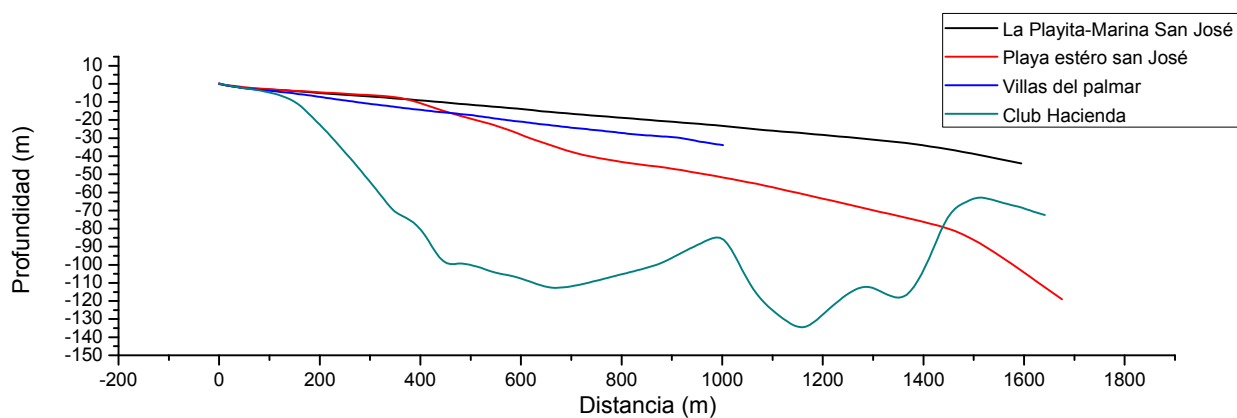
Figura 6. Perfiles batimétricos de la línea de costa hacia mar adentro, en el destino turístico Los Cabos
