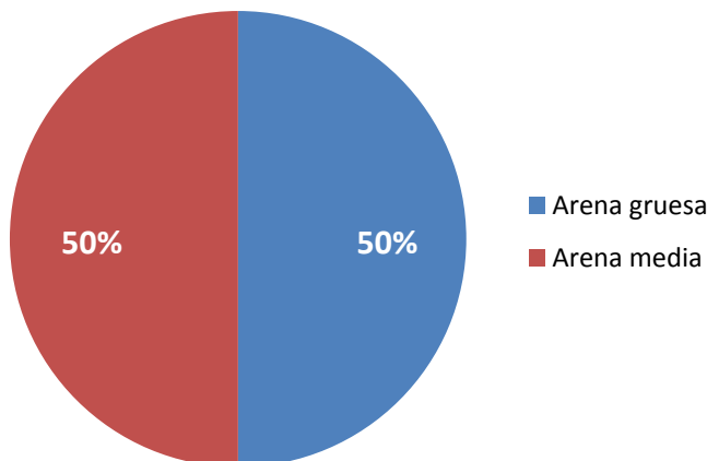
Figura 9. Tipo de sedimentos en playas de San José del Cabo, Los Cabos
