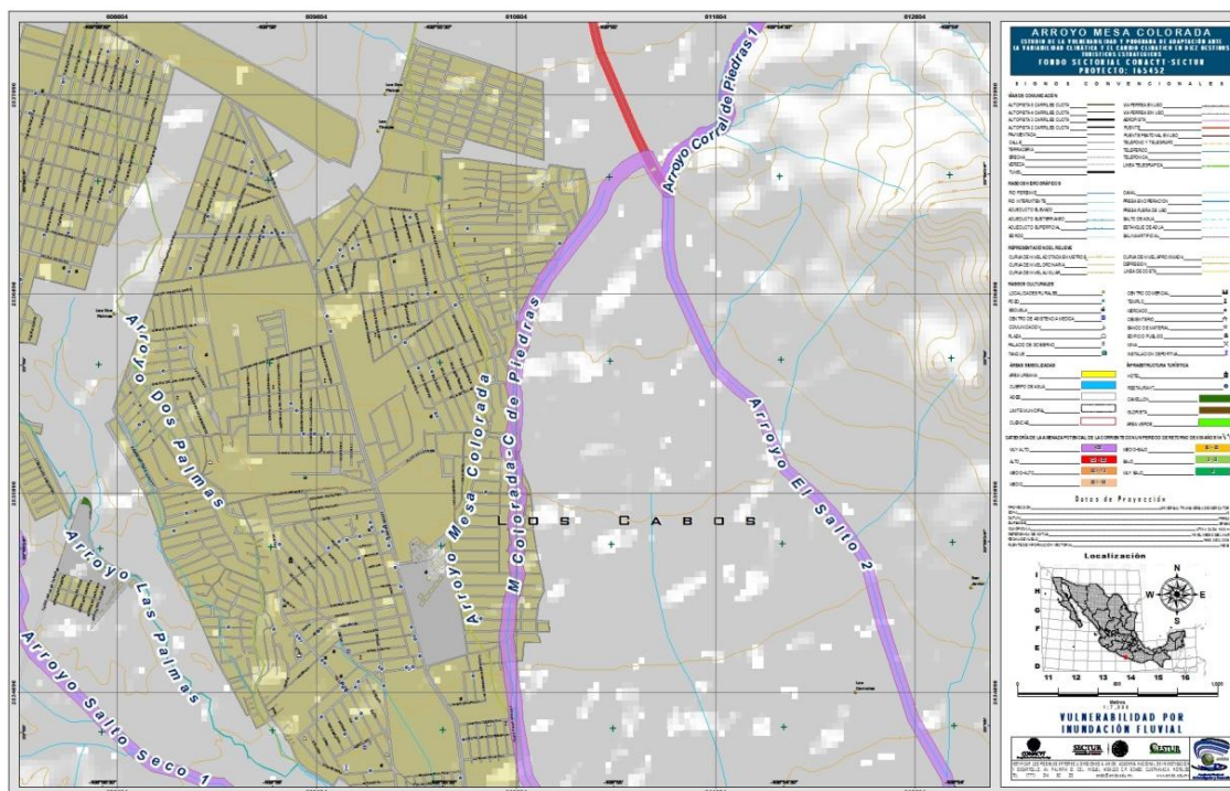
Figura 29. Áreas de inundación fluvial del río Mesa Colorada en el destino turístico de Los Cabos
