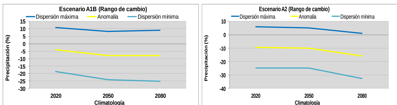
Figura 12. Rango de cambio en la Precipitación Media Anual (%) en Los Cabos
