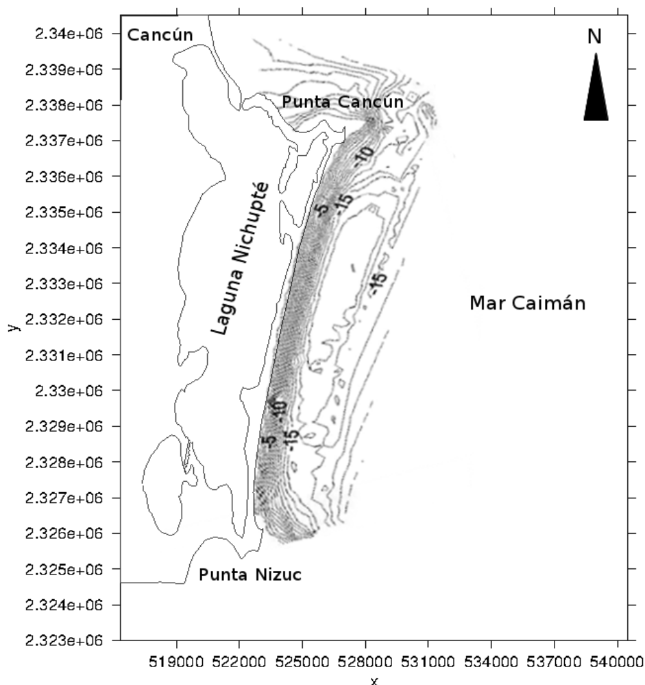
Figura 8. Batimetría del destino turístico de Cancún
