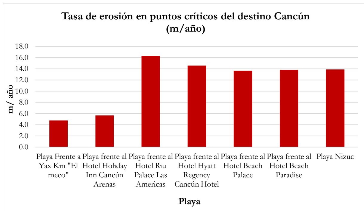
Figura 15. Tasa de erosión en puntos críticos del destino turístico de Cancún
