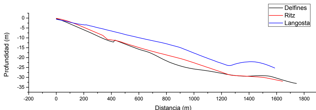
Figura 9. Perfiles batimétricos de la línea de costa hacia mar adentro, en el destino turístico de Cancún
