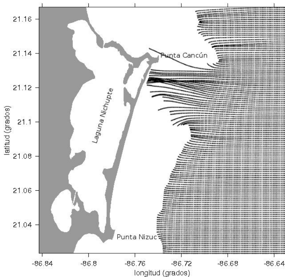
Figura 22. Comportamiento de ortogonales de oleaje en Cancún, provenientes de la dirección E, 6 segundos
