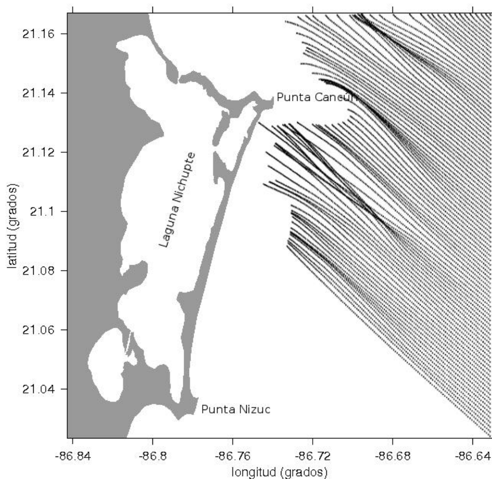
Figura 21. Comportamiento de ortogonales de oleaje en Cancún, provenientes de la dirección SE, 12 segundos
