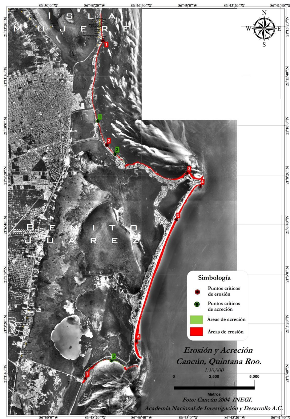
Figura 14. Puntos críticos de mayor erosión y acreción en el destino turístico de Cancún
