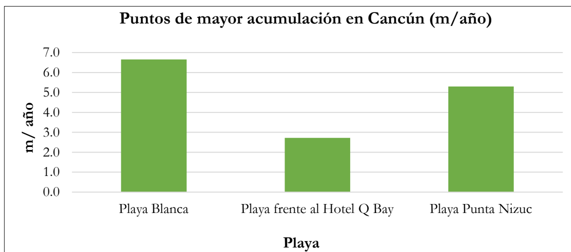
Figura 16. Tasa de acreción en puntos de mayor acumulación del destino turístico de Cancún
