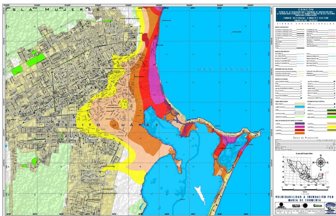
Figura 18. Zonas vulnerables a inundación por marea de tormenta en el destino turístico Cancún
